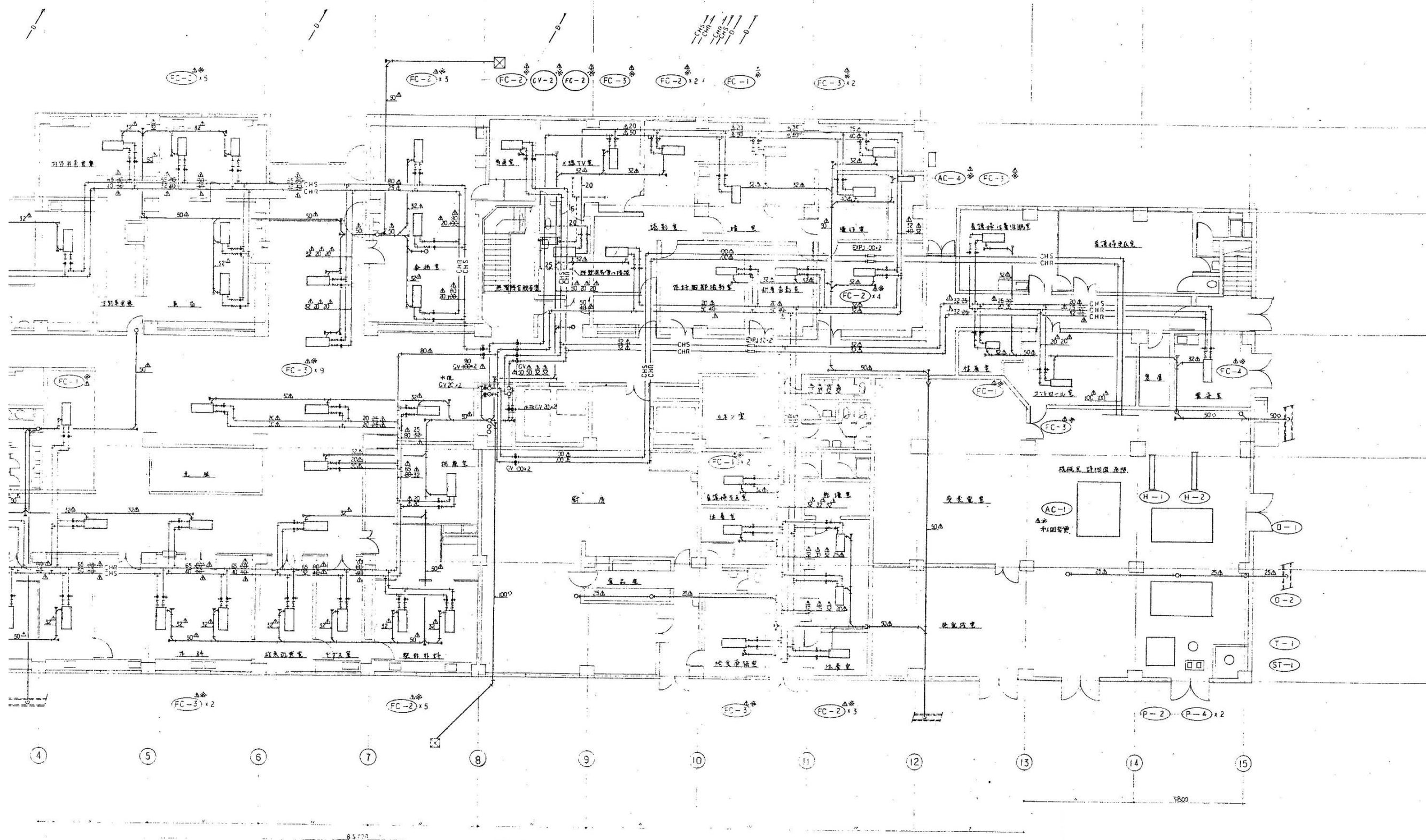
1階平面図 配管 S=1/100
